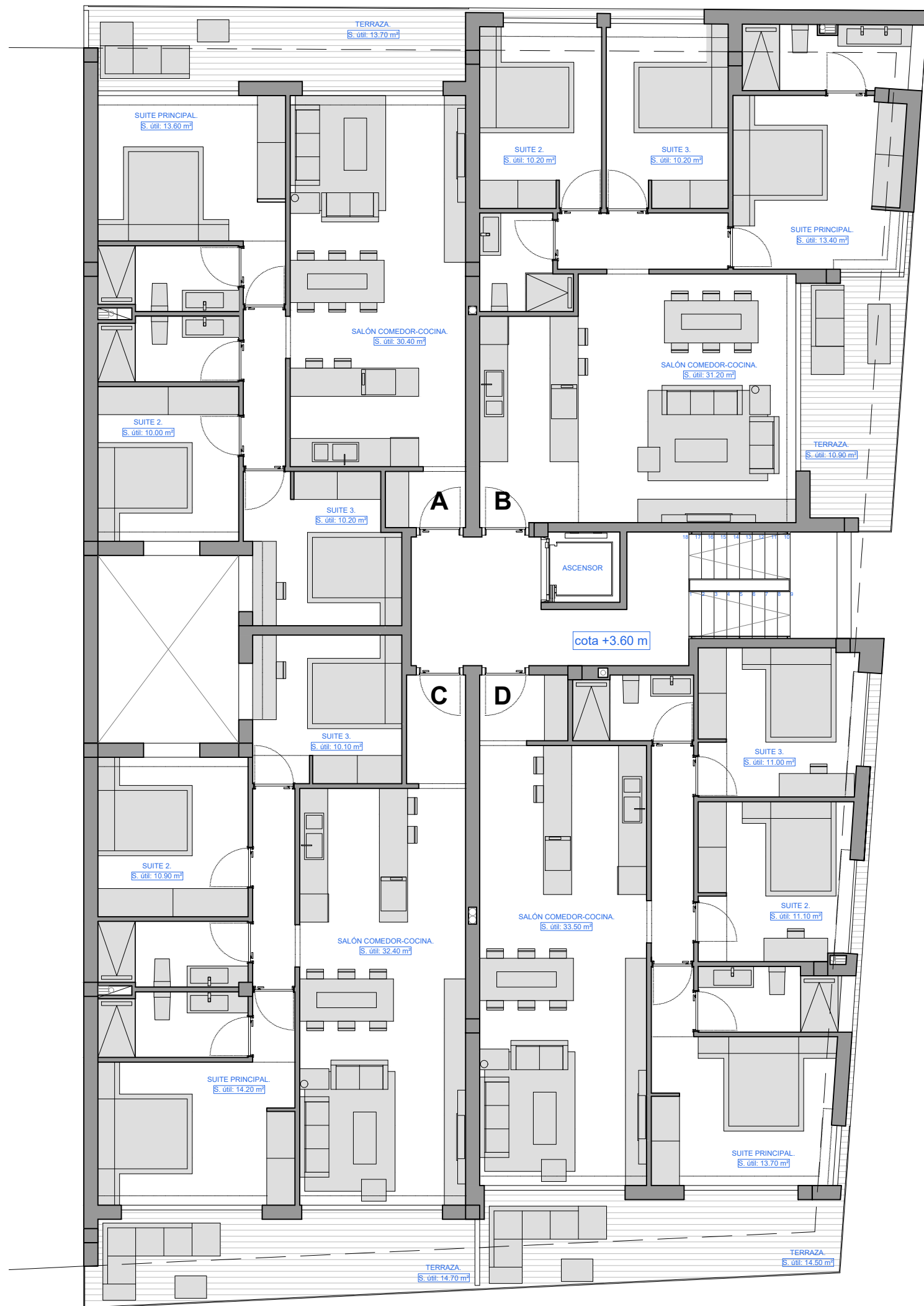
PLANTA PRIMERA. Superficie Construida Total: 390.30 m 2 Superficie Terrazas Cubiertas: 53.80 m 2
